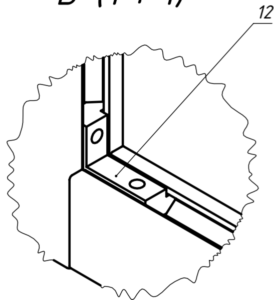
D (1 : 1)
