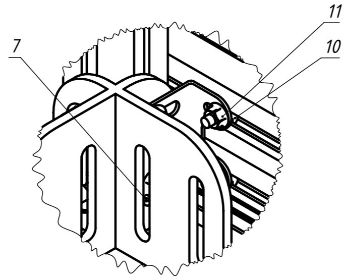
E (1 : 2)
