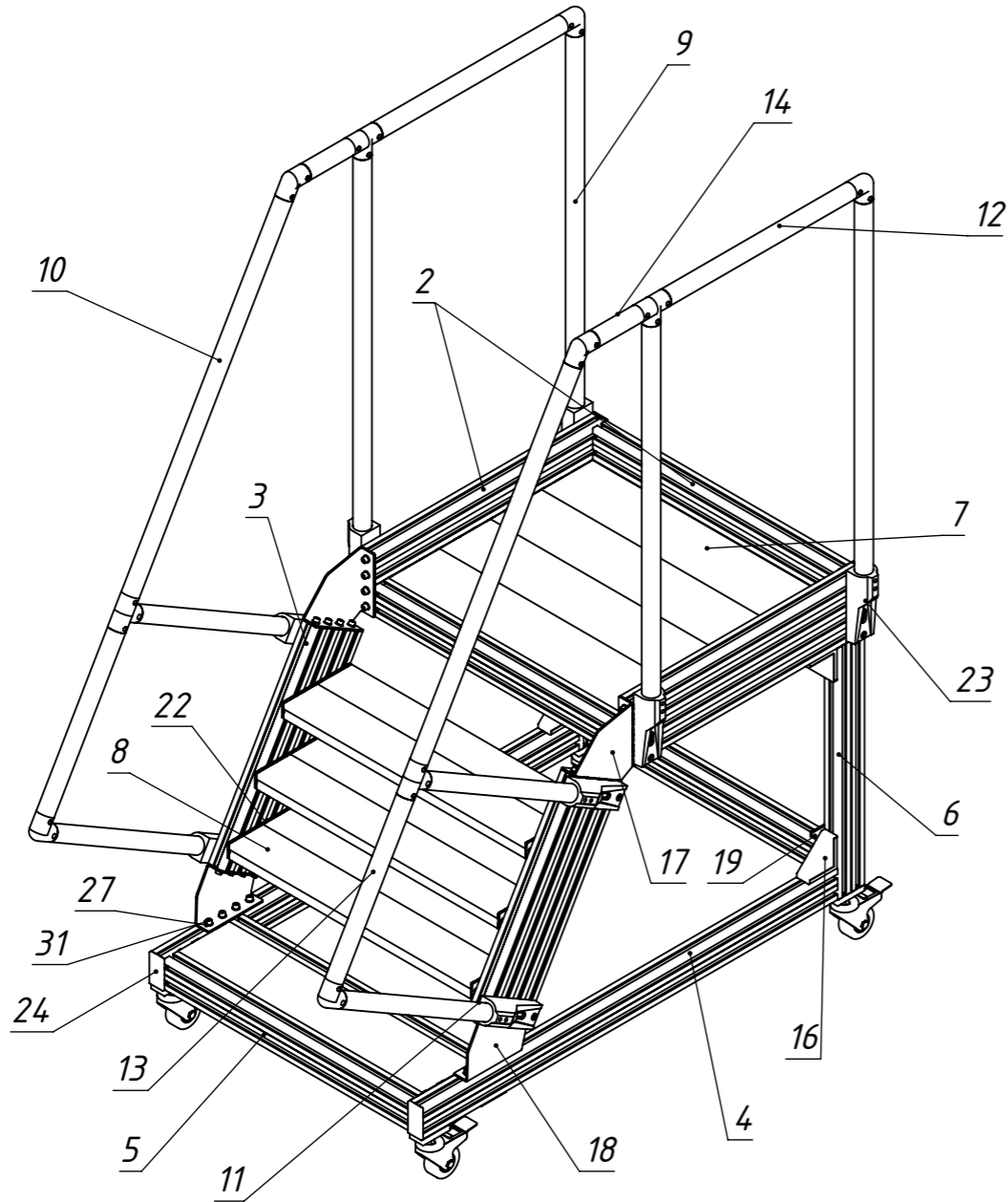
A (1 : 5)
